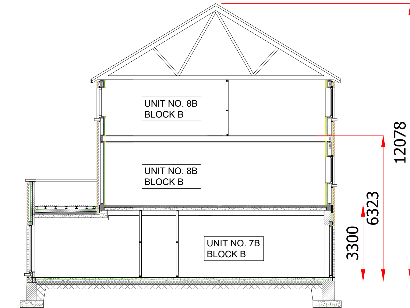
Section A-A
